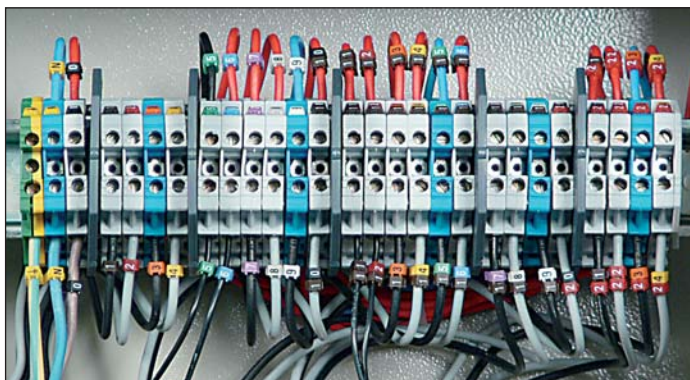
Bornier intégré dans l'armoire
